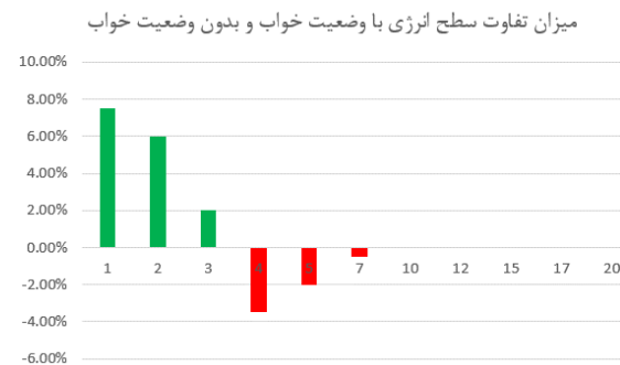
شکل ۱۱: میزان تفاوت سطح انرژی با وضعیت خواب و بدون وضعیت خواب با توجه به تعداد گره های متصل به سرخوشه
